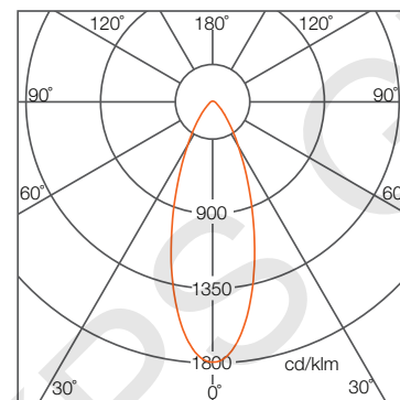
White, 36°
