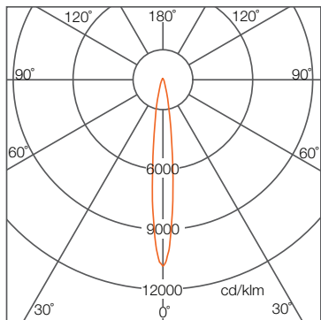
White, 11°
